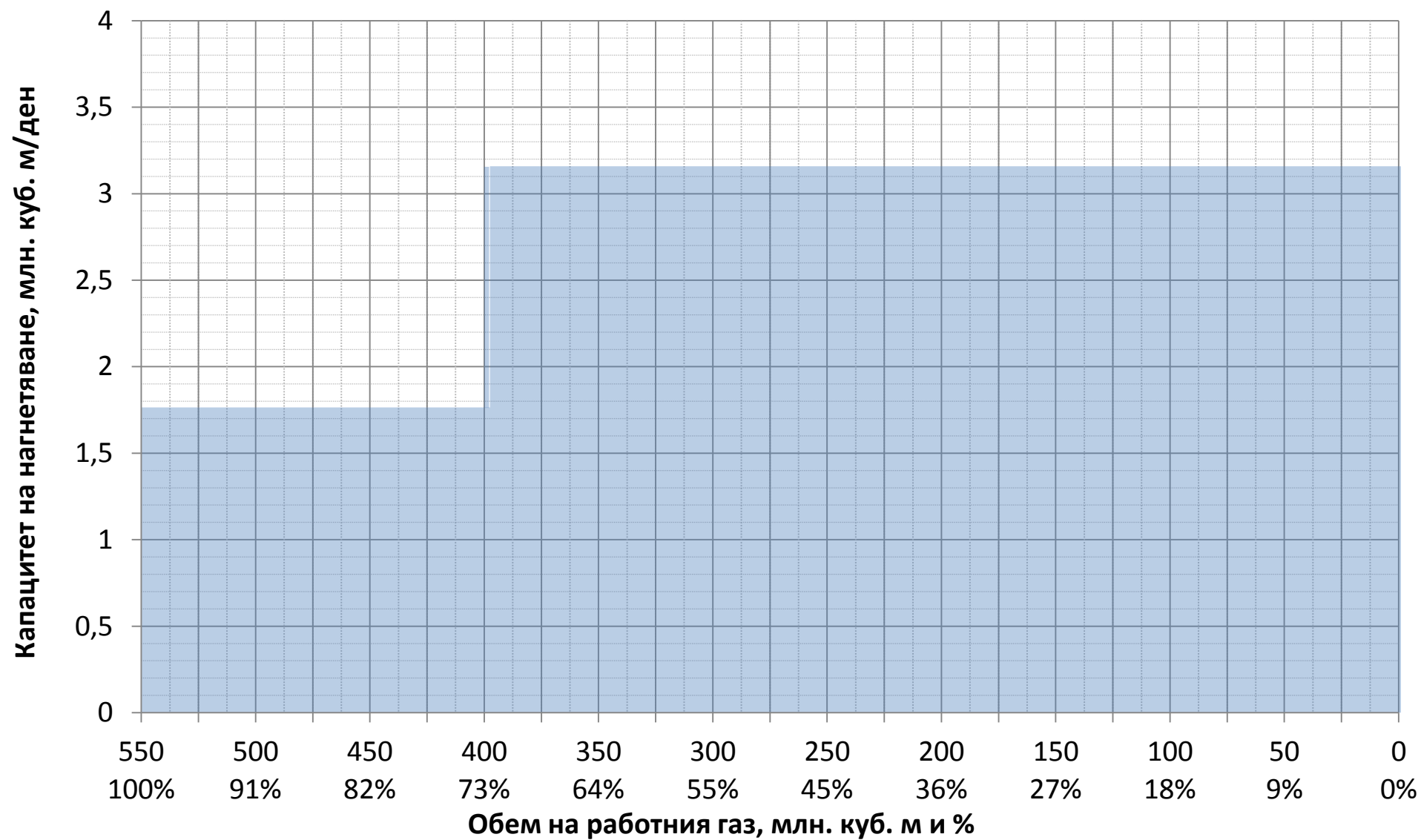
Крива на капацитета на нагнетяване на ПГХ Чирен за газова година 2018-2019, млн. куб. м
